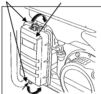
ELEMENTO DO FILTRO DE AR
