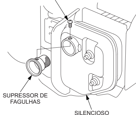
PARAFUSO AUTOTARRAXANTE 3x6 mm
