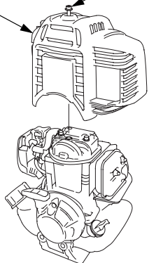
TAMPA SUPERIOR PARAFUSO SEXTAVADO INTERNO, 5 mm
