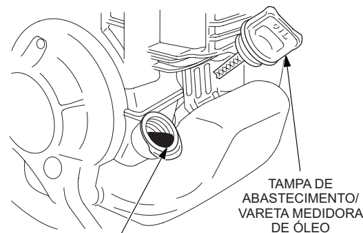
ORIFÍCIO DE ABASTECIMENTO DE ÓLEO (borda inferior)
