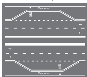
Marca delimitadora para parada de ônibus feita em reentrância da calçada
