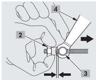
Freio Dianteiro (BIZ125 KS • ES)
