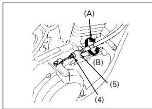
(4) Contraporca (5) Porca de ajuste (A) Aumenta a folga (B) Diminui a folga
