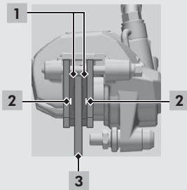
Freio dianteiro
