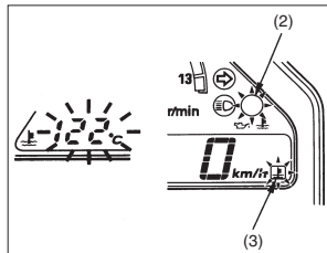
(2) Luz de advertência de falha (3) Indicador de advertência da temperatura do líquido de arrefecimento
