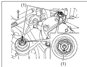
(1) Ajustador da ação do amortecedor
