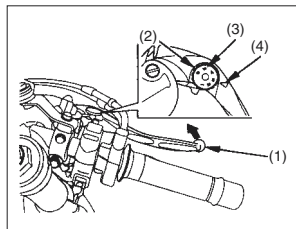
(1) Alavanca do freio (2) Ajustador (3) Números (4) Seta
