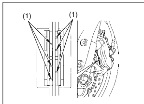
(1) Ranhura indicadora de desgaste
