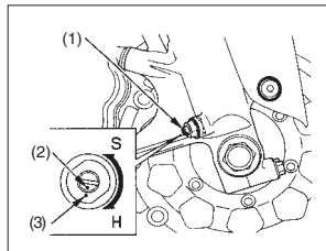
(1) Ajustador do amortecedor (2) Marca (3) Marca de referência
