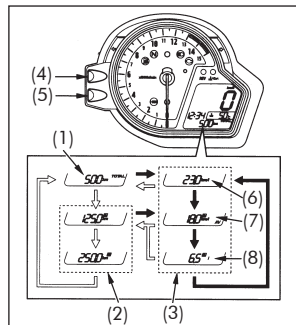
(1) Indicador do amortecedor de direção eletrônico Honda
