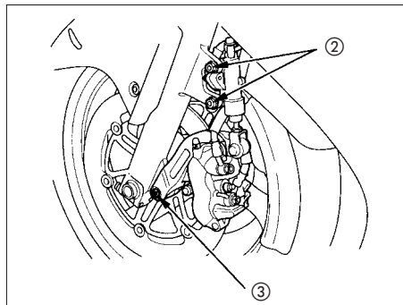
(2) Parafusos Allen A
