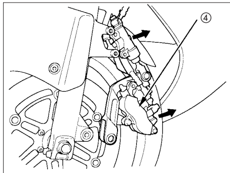
(4) Conjunto do caliper esquerdo
