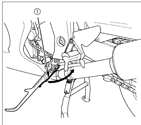
(1) Mola do cavalete lateral
