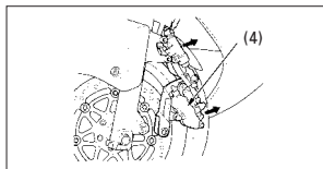
(4) Conjunto do câliper esquerdo
