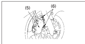
(5) Conjunto do câliper direito (6) Parafusos de fixação
