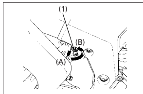
(1) Parafuso de aceleração (A) Aumenta a rotação (B) Diminui a rotação
