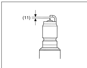
(11) Folga entre os eletrodos
