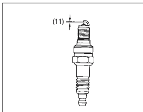
(11) Folga dos eletrodos
