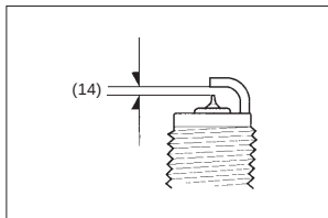
(14) Folga entre os eletrodos
