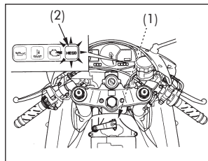
(1) Amortecedor de direção eletrônico Honda (2) Indicador do amortecedor de direção eletrônico Honda
