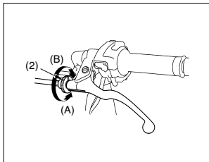
(2) Ajustador do cabo da embreagem (A) Aumenta a folga (B) Diminui a folga
