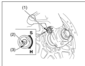
(1) Ajustador do amortecedor (2) Marca (3) Marca de referência
