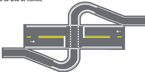
Marcação de cruzamento rodociclovitário
