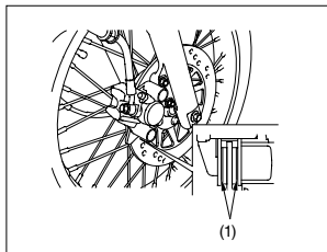
(1) Ranhura indicadora de desgaste
