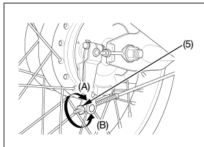
(5) Porca de ajuste (A) Diminui a folga (B) Aumenta a folga
