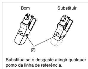
(2) Linha de referência
