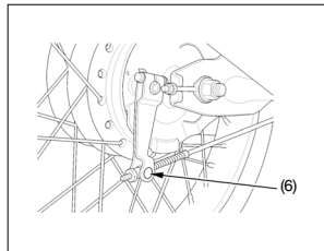
(6) Articulação do braço do freio
