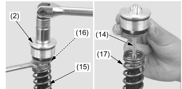
(2) PARAFUSO SUPERIOR DO GARFO DA SUSPENSÃO (14) HASTE DA AGULHA DO AJUSTADOR (15) HASTE DO PISTÃO (16) CONTRAPORCA (17) MOLA DO GARFO DA SUSPENSÃO
