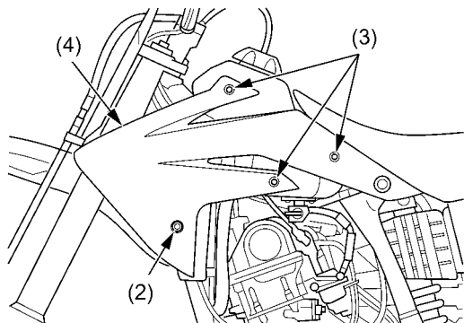
(2) PARAFUSO/ESPAÇADOR A DO PROTETOR (3) PARAFUSOS B DO PROTETOR (4) PROTETOR
