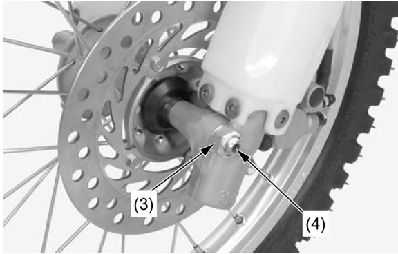
(3) PORCA DO EIXO DIANTEIRO (4) EIXO DIANTEIRO
