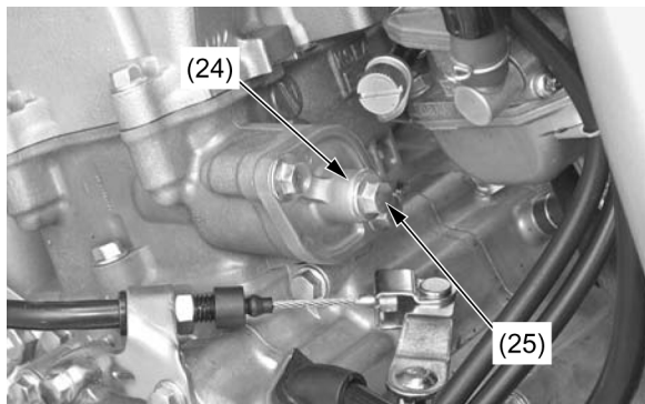
(24) ARRUELA DE VEDAÇÃO
