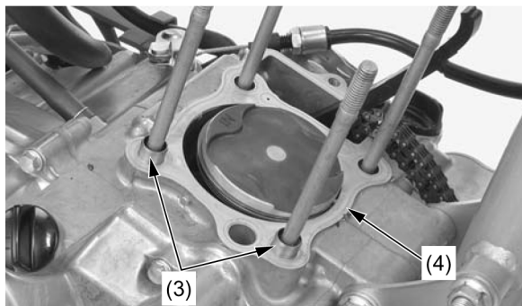
(3) PINOS-GUIAS (4) JUNTA DO CILINDRO
