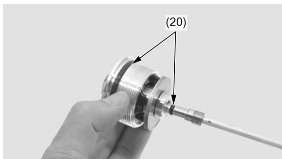
(20) ANÉIS DE VEDAÇÃO
