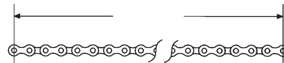
MEDIDA ENTRE 21 PINOS (20 ELOS)
