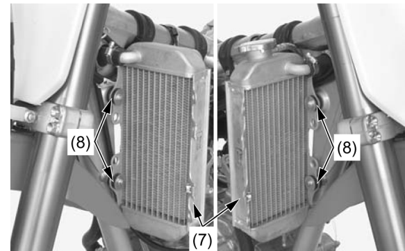
(7) RADIADORES (8) PARAFUSOS/ARRUELAS DE FIXAÇÃO DOS RADIADORES
