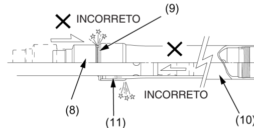
(8) CILINDRO INTERNO (9) RETENTOR DE PÓ (10) CILINDRO EXTERNO (11) BUCHA DA GUIA
