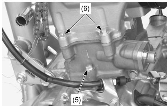
(5) PARAFUSO DO CILINDRO (6) PARAFUSOS DO CABEÇOTE
