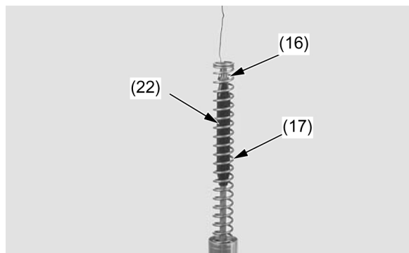
(16) CONTRAPORCA (17) MOLA DO GARFO DA SUSPENSÃO (22) GUIA DA MOLA
