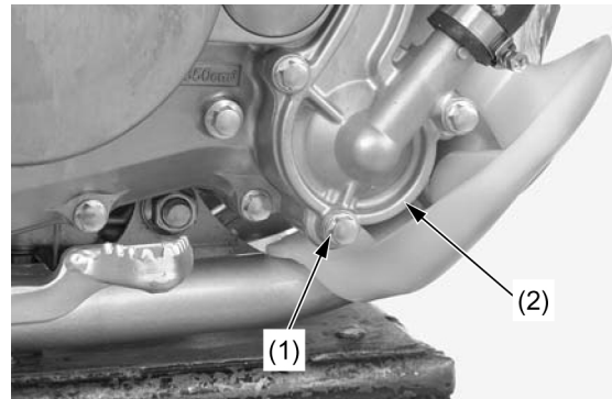
(1) PARAFUSO DE DRENAGEM DO LÍQUIDO DE ARREFECIMENTO/ARRUELA DE VEDAÇÃO (2) BOMBA DE ÁGUA
