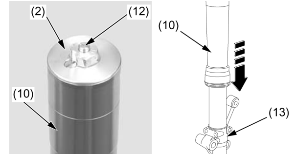
(2) PARAFUSO SUPERIOR DO GARFO DA SUSPENSÃO (10) CILINDRO EXTERNO (12) PARAFUSO DE AJUSTE (13) CILINDRO INTERNO, EXTREMIDADE INFERIOR
