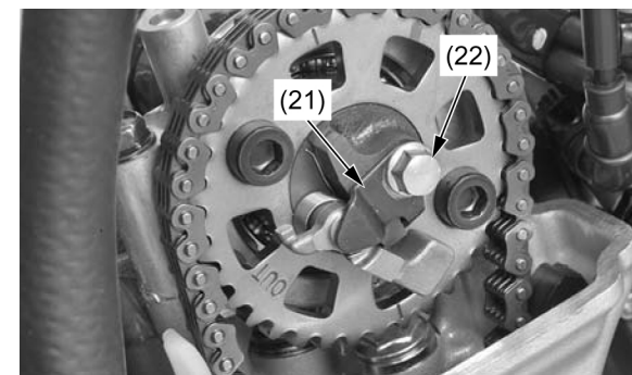
(21) PLACA LIMITADORA (22) PARAFUSO
