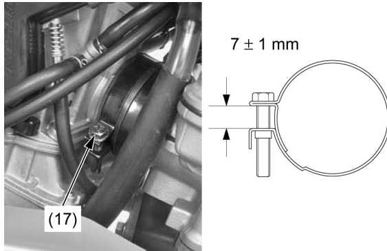
(17) PARAFUSO DA BRAÇADEIRA DO ISOLANTE
