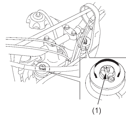
(1) AJUSTADOR DE AMORTECIMENTO
