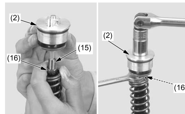
(2) PARAFUSO SUPERIOR DO GARFO DA SUSPENSÃO (15) HASTE DO PISTÃO (16) CONTRAPORCA
