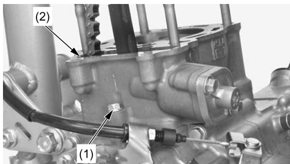
(1) PARAFUSO DO CILINDRO (2) CILINDRO
