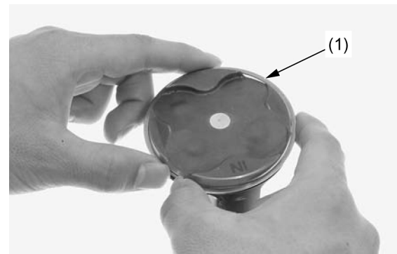
(1) ANEL DO PISTÃO
