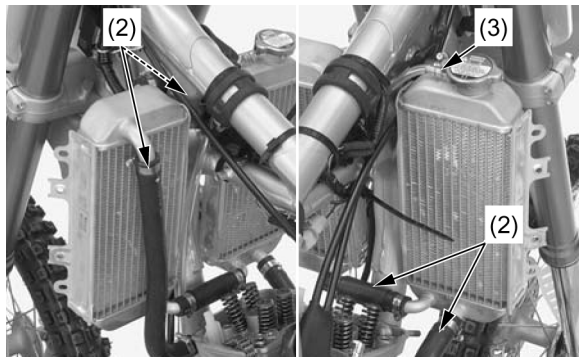
(2) MANGUEIRAS DE ÁGUA (3) MANGUEIRA-SIFÃO DO RADIADOR
