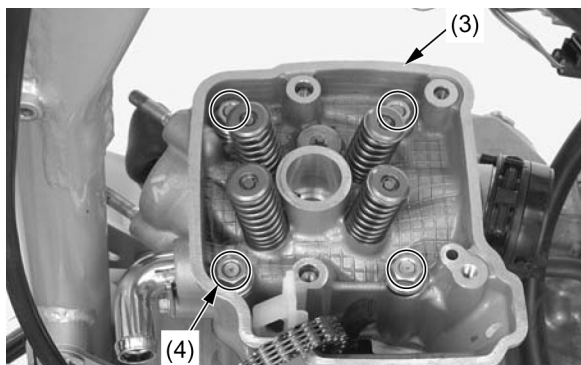
(3) CABEÇOTE (4) PORCAS/ARRUELAS DO CABEÇOTE
