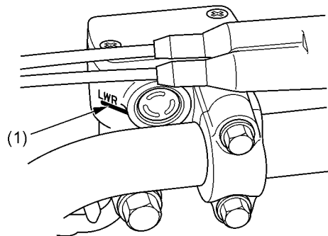
(1) MARCA LWR (INFERIOR)
