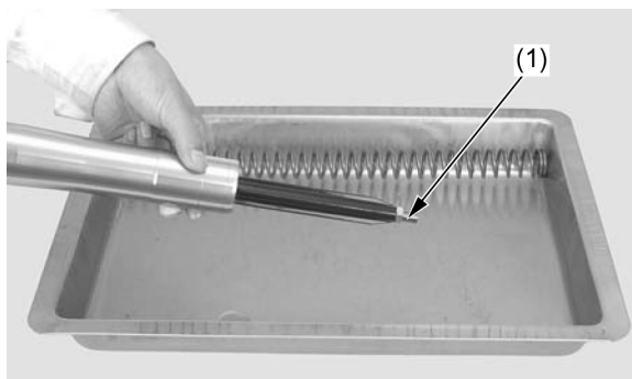
(1) HASTE DO PISTÃO
