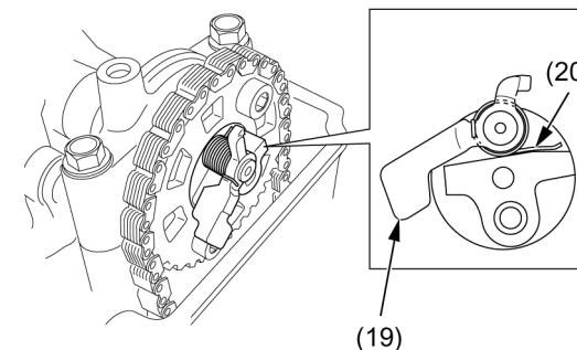
(19) DESCOMPRESSOR (20) MOLA DE RETORNO
