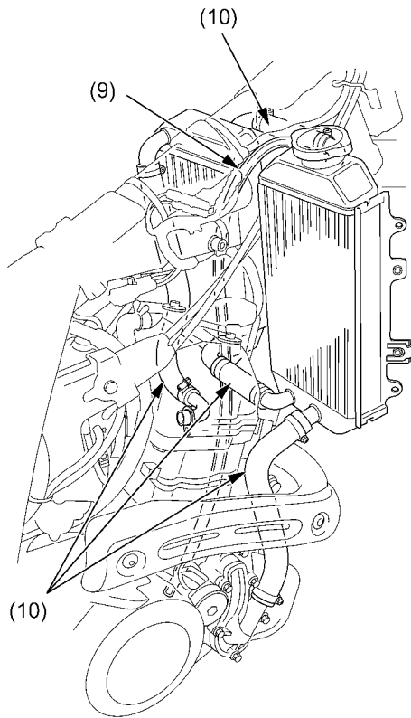
(9) MANGUEIRA-SIFÃO DO RADIADOR (10) MANGUEIRAS DE ÁGUA
