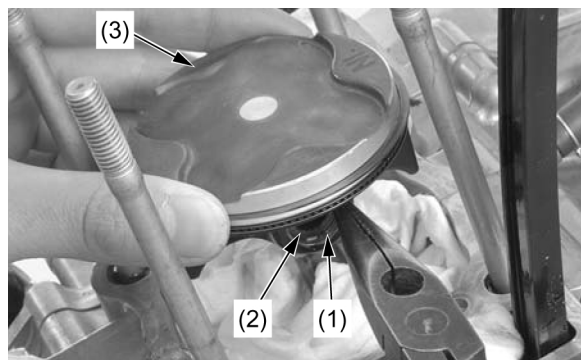
(1) PRESILHA DO PINO DO PISTÃO (2) PINO DO PISTÃO (3) PISTÃO
