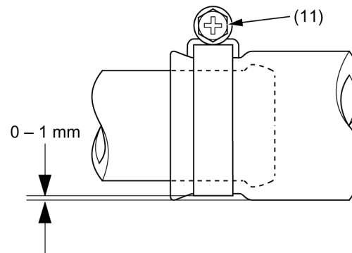
(11) PARAFUSO DA BRAÇADEIRA DA MANGUEIRA
