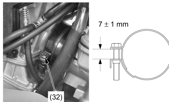
(32) PARAFUSO DA BRAÇADEIRA DO ISOLANTE
