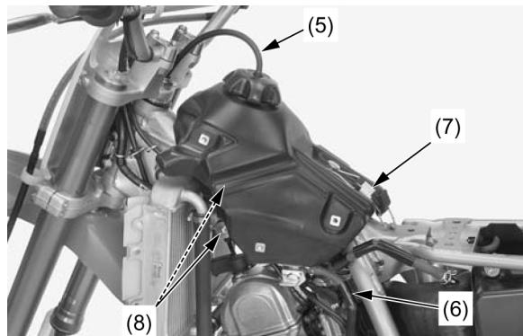
(5) TUBO DE RESPIRO (6) LINHA DE COMBUSTÍVEL (7) CINTA DO TANQUE DE COMBUSTÍVEL (8) PARAFUSOS/ARRUELAS DO TANQUE DE COMBUSTÍVEL
