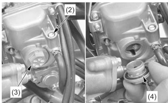
(2) PARAFUSO DE DRENAGEM (3) BUJÃO DA CUBA DA BÓIA (4) ANEL DE VEDAÇÃO DO BUJÃO DA CUBA DA BÓIA
