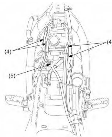
(4) MANGUEIRAS DE VENTILAÇÃO (5) MANGUEIRA-SIFÃO
