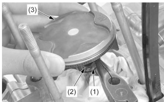
(1) PRESILHA DO PINO DO PISTÃO (2) PINO DO PISTÃO (3) PISTÃO
