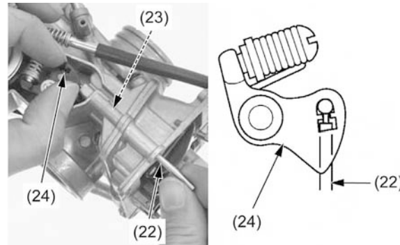
(22) HASTE DA BOMBA (23) PASSAGEM DA HASTE (24) ALAVANCA DE CONEXÃO
