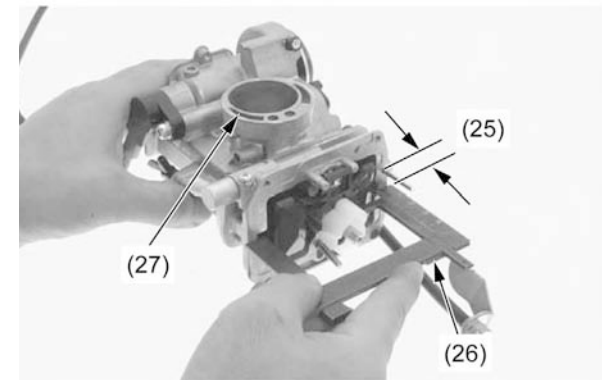
(25) NÍVEL DA BÓIA (26) MEDIDOR DE NÍVEL DA BÓIA (27) ADMISSÃO DO CARBURADOR
