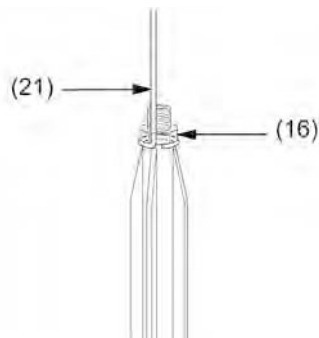
(16) CONTRAPORCA (21) ARAME
