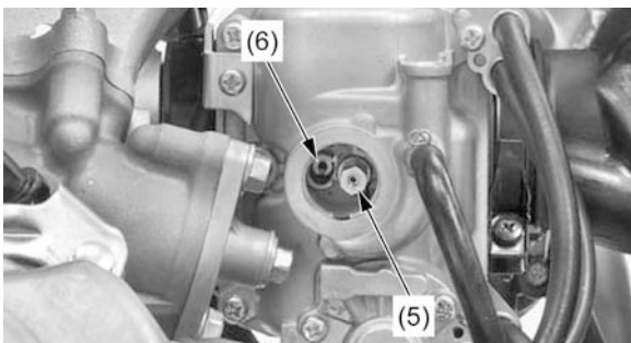
(5) GICLÊ PRINCIPAL (6) GICLÊ DE MARCHA-LENTA
