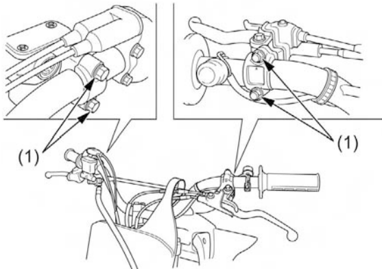
(1) PARAFUSOS DE FIXAÇÃO DA ALAVANCA DE CONTROLE
