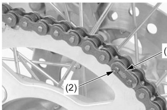
(1) PRESILHA DE RETENÇÃO DO ELO-MESTRE (2) ELO-MESTRE
