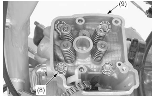
(8) PORCAS/ARRUELAS DO CABEÇOTE (9) CABEÇOTE
