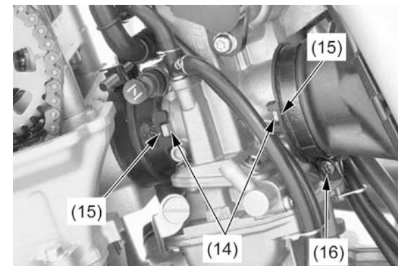
(14) LINGUETAS (15) RANHURAS (16) PARAFUSO DA BRAÇADEIRA DO TUBO DE CONEXÃO
