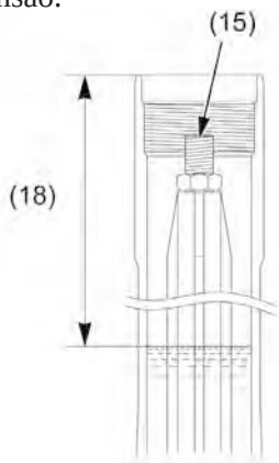
(15) HASTE DO PISTÃO (18) NÍVEL DE FLUIDO
