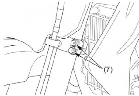
(7) PARAFUSOS DE FIXAÇÃO DA MESA INFERIOR DO GARFO DA SUSPENSÃO
