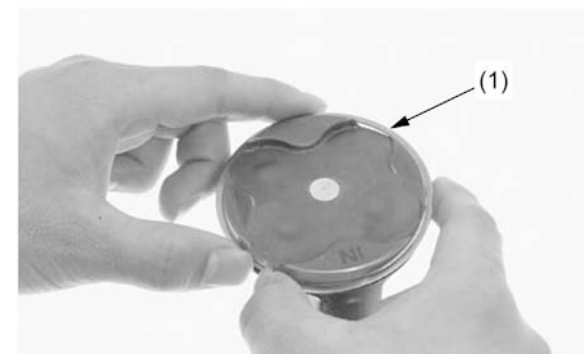
(1) ANEL DO PISTÃO
