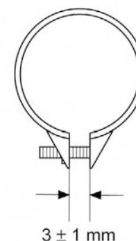
(14) LINGUETAS (15) RANHURAS (16) PARAFUSO DA BRAÇADEIRA DO TUBO DE CONEXÃO
