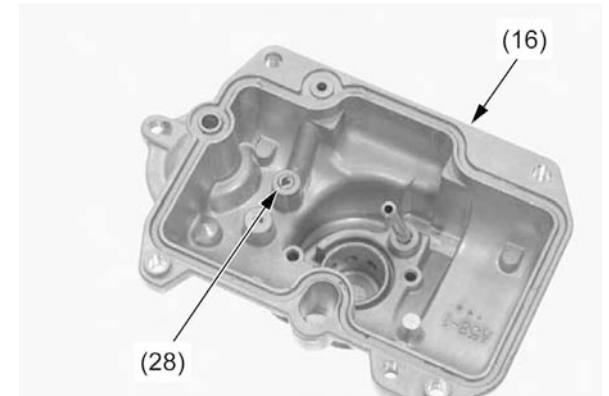
(16) CUBA DA BÓIA (28) GICLÊ AUXILIAR
