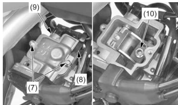
(7) PARAFUSOS DA TAMPA DO CARBURADOR (8) PRESILHA DO CABO (9) TAMPA DO CARBURADOR (10) CONJUNTO DA AGULHA/PULVERIZADOR
