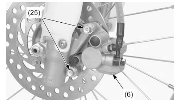
(6) CÁLIPER DO FREIO (25) PARAFUSOS DE FIXAÇÃO DO CÁLIPER DO FREIO
