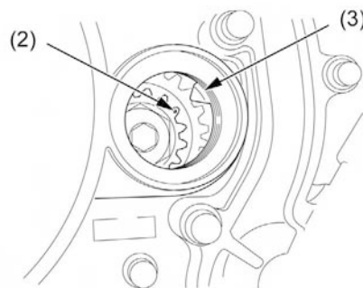
(2) MARCA GRAVADA
