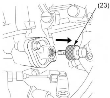
(23) LIMITADOR DO TENSOR
