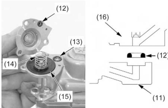
(11) TAMPA DA BOMBA DE ACELERAÇÃO (12) VEDADOR (13) ANEL DE VEDAÇÃO (14) MOLLA (15) DIAFRAGMA (16) CUBA DA BÓIA
