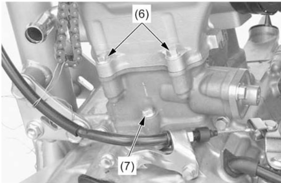
(6) PARAFUSOS DO CABEÇOTE (7) PARAFUSO DO CILINDRO
