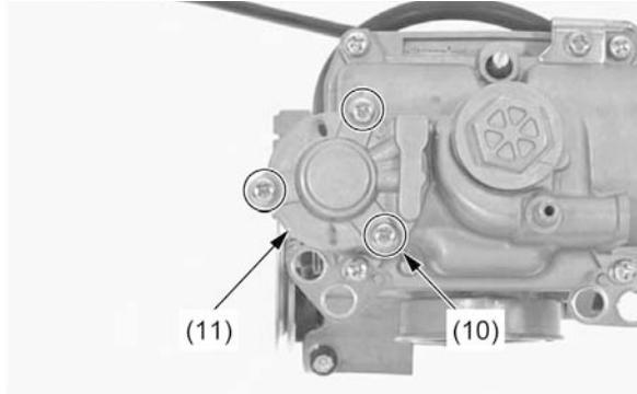
(10) PARAFUSOS DA TAMPA DA BOMBA DE ACELERAÇÃO (11) TAMPA DA BOMBA DE ACELERAÇÃO
