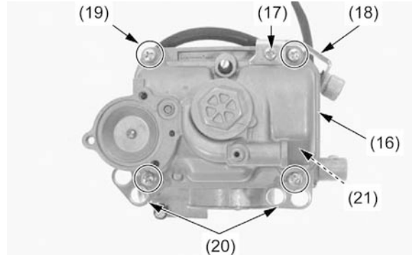
(16) CUBA DA BÓIA (17) PARAFUSOS DO SUPORTE (18) SUPORTE DO PARAFUSO DE ACELERAÇÃO (19) PARAFUSOS DA CUBA DA BÓIA (20) GUIAS DA MANGUEIRA (21) ANEL DE VEDAÇÃO
