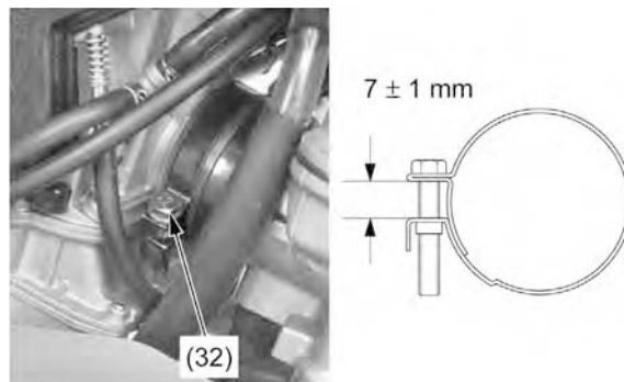
(32) PARAFUSO DA BRAÇADEIRA DO ISOLANTE
