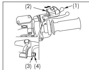
(1) Alavanca do freio dianteiro (2) Protetor de borracha (3) Contraporca (4) Ajustador
