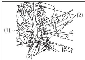
(1) Rolamentos do braço oscilante (2) Fixadores
