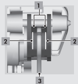
Freio dianteiro
