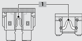
1. Fusível queimado
