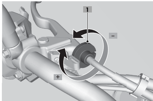
1. Ajustador superior do cabo da embreagem
