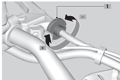
1. Ajustador superior do cabo da embreagem
