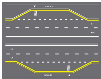
MARCA DELIMITADORA PARA PARADA DE ÔNIBUS FEITA EM REENTRÂNCIA DA CALÇADA
