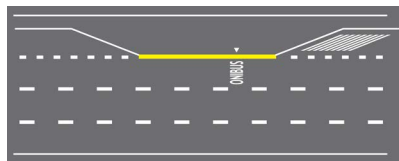
MARCA DELIMITADORA PARA PARADA DE ÔNIBUS EM FAIXA DE TRÂNSITO COM AVANÇO DE CALÇADA NA FAIXA DE ESTACIONAMENTO
