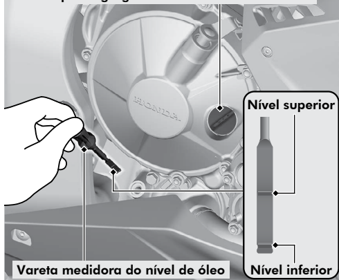
Tampa do gargalo de abastecimento de óleo
