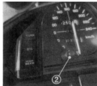
(2) Botão de "zeragem" do hodômetro parcial
