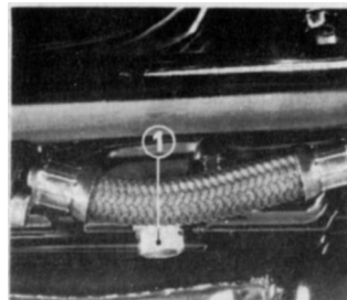
(1) Bujão de drenagem do motor
