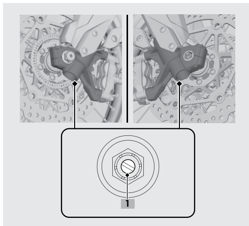
1. Ajustador
