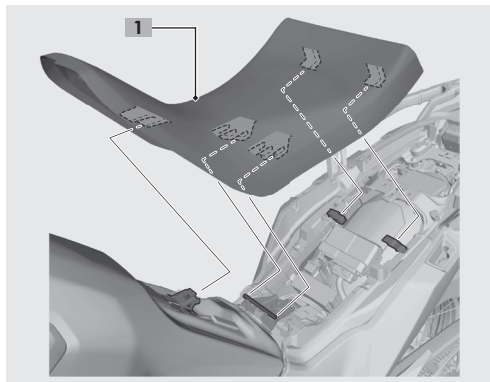
1. Assento dianteiro
