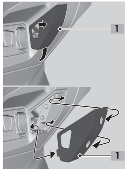
1. Tampa dianteira
