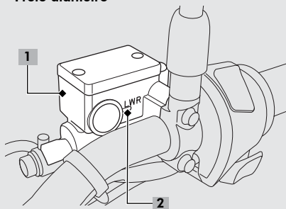
Freio dianteiro
