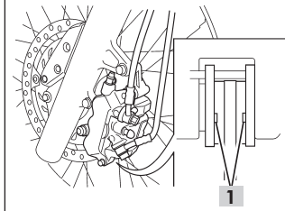
Freio dianteiro (XRE300A)
