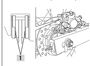
Freio traseiro (XRE300A)
