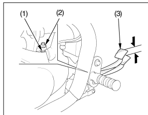
(1) Parafuso limitador (2) Contraporca (3) Pedal do freio traseiro
